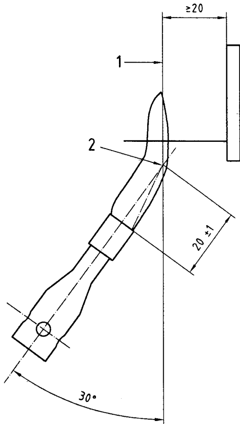
b) Bottom edge ignition
